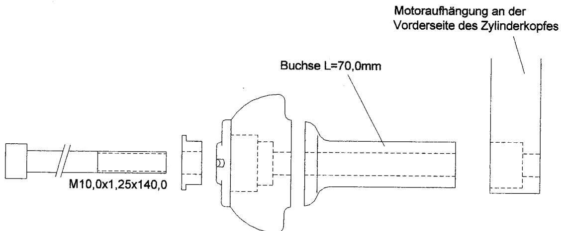
Montageteile links
