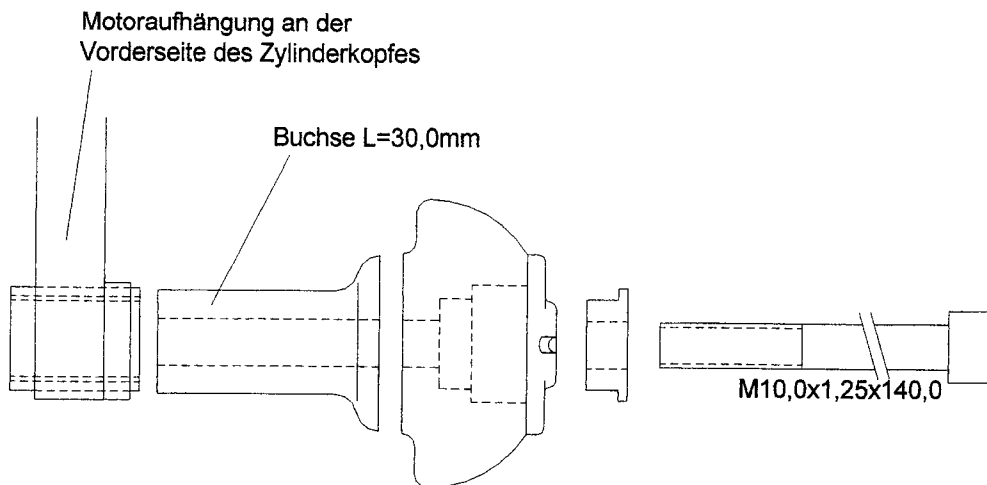
Montageteile rechts
