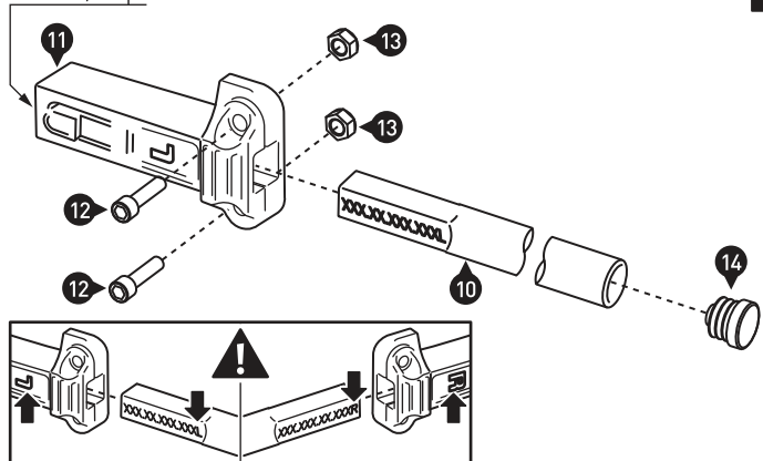
Lasche / Clip
