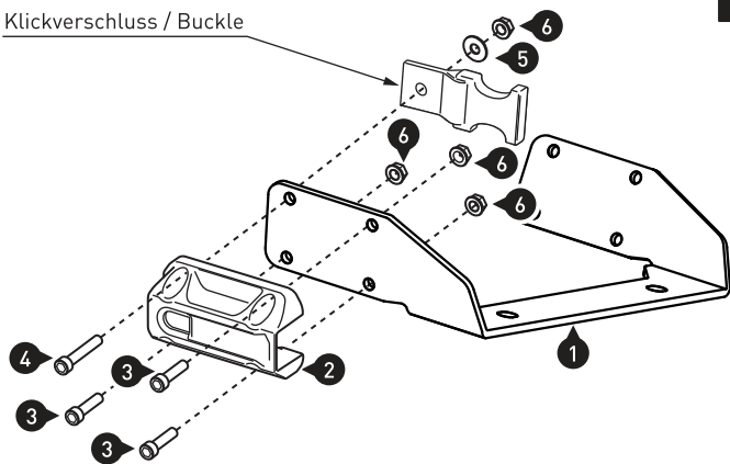
Klickverschluss / Buckle
