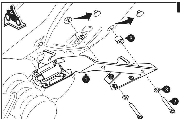
Lasche / Clip
